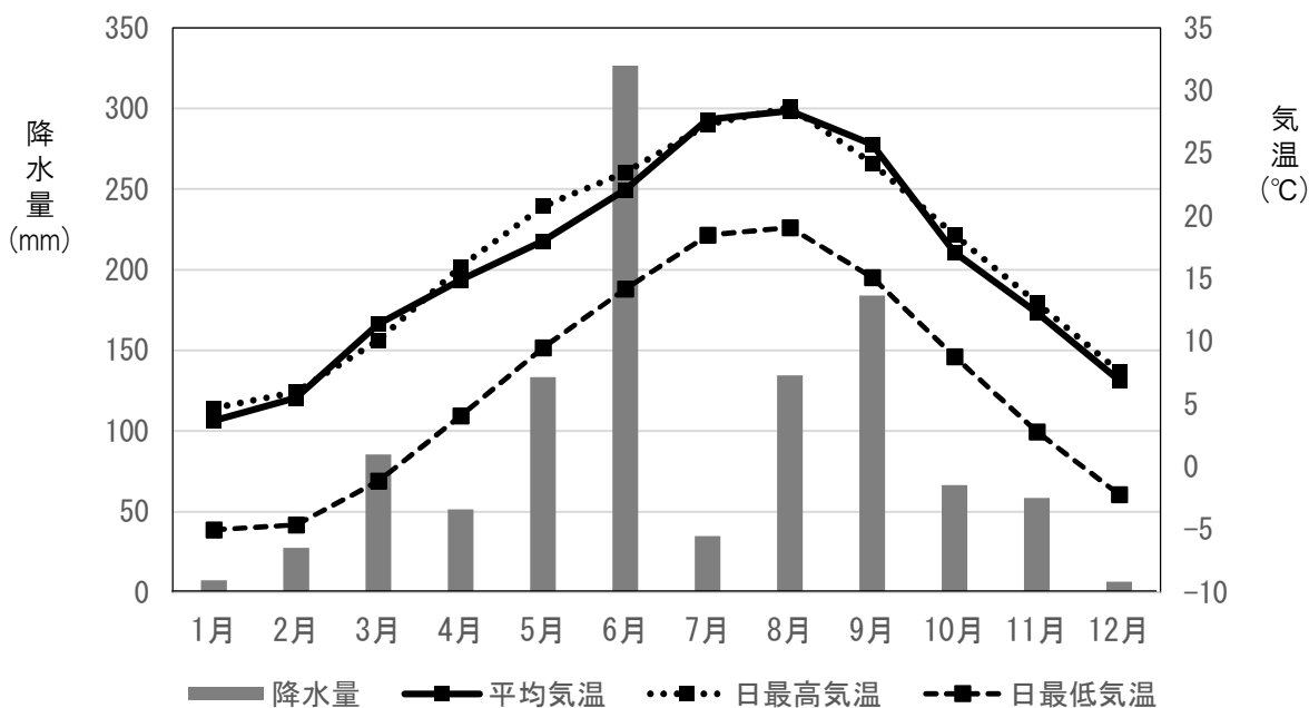
【令和5年の降水量・月平均気温（青梅観測点）】
