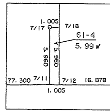
拡大図S=1:250
