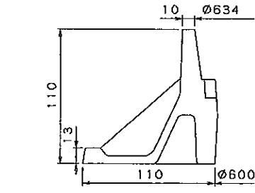
フレーム一般断面図
