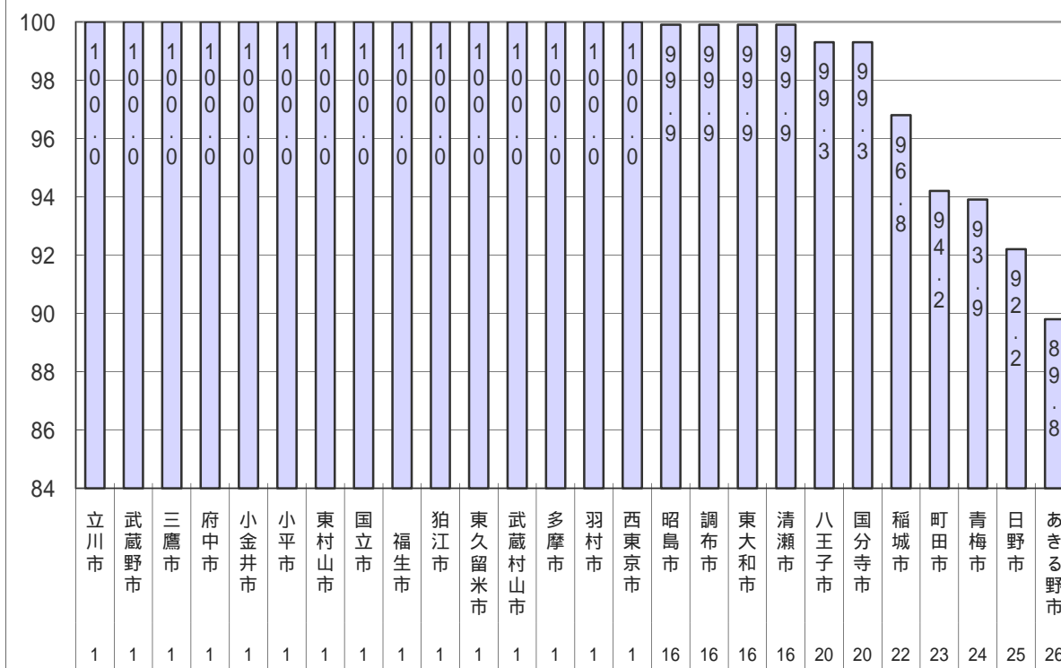
4-2. グラフ 下水道普及率 (平成22年4月1日) 単位: %
