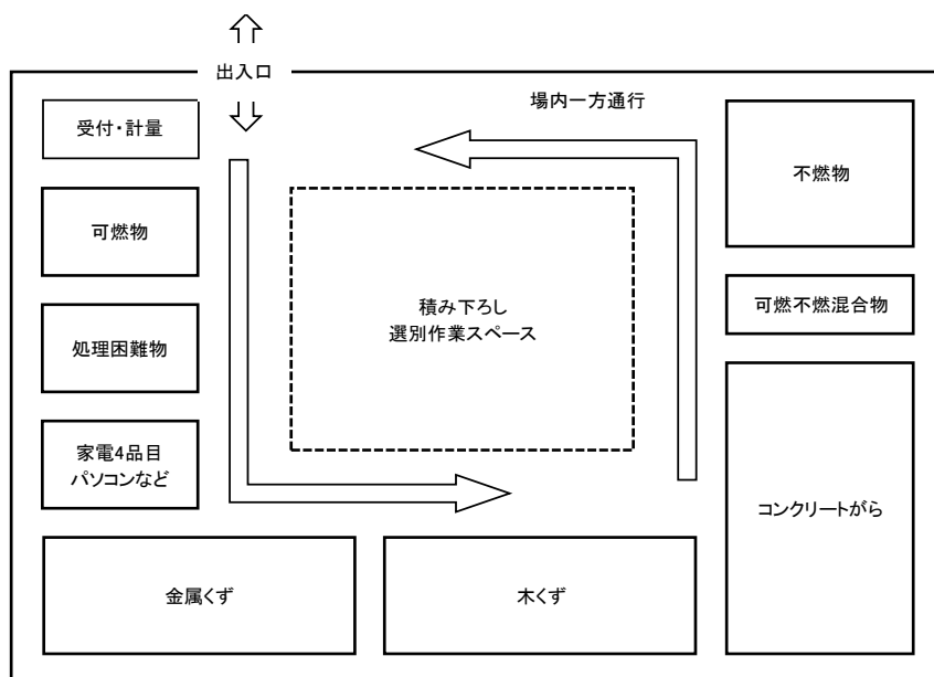
図7-5-3 一次仮置場のレイアウト例
