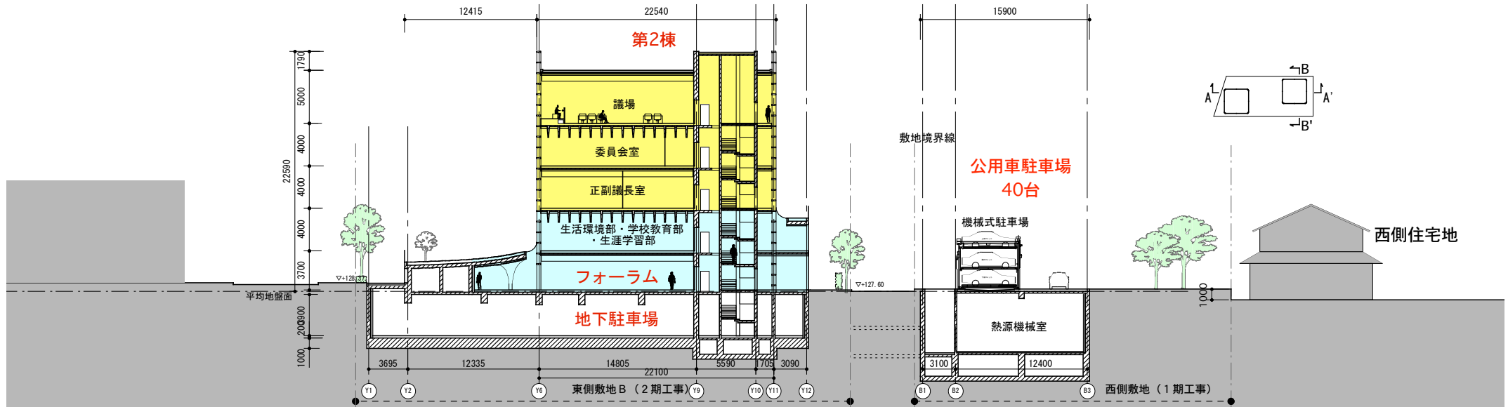
B-B' 断面図
