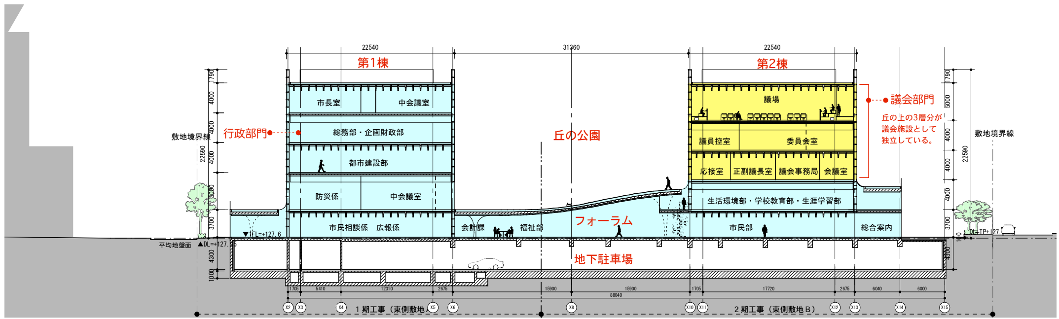
A-A' 断面図
