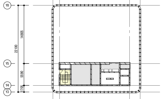
塔屋階平面図
